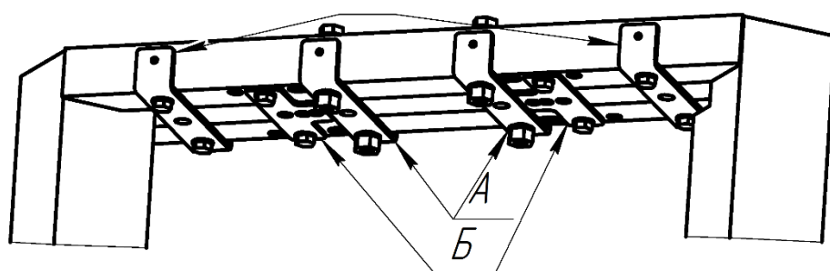
Скоба №3.
