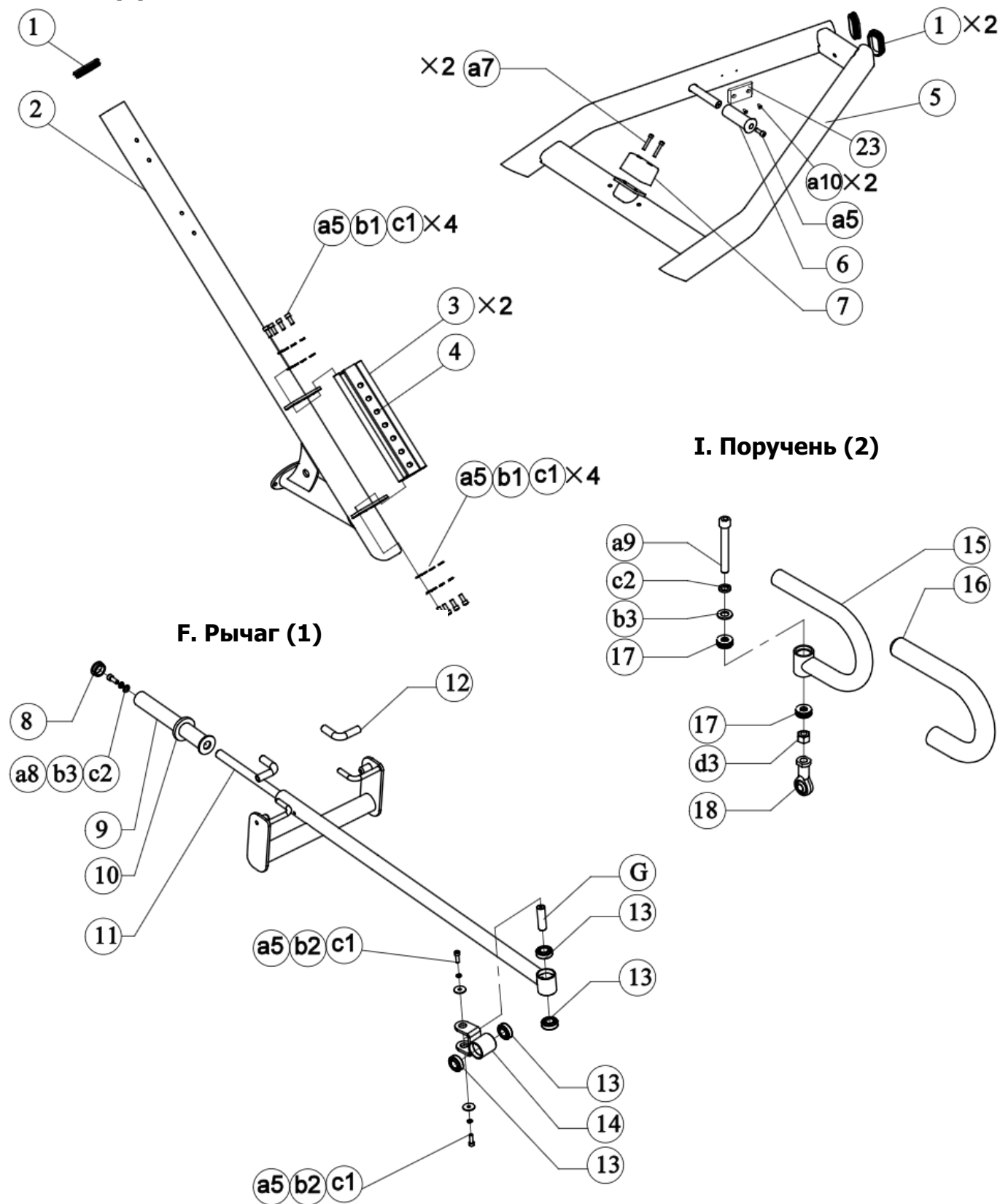
В. Основная рама в сборке (1)
